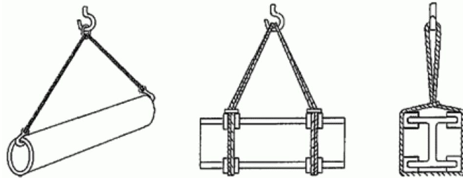
Строп с крюками для металлической трубы
