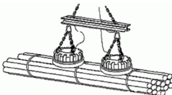
Грузоподъемные электромагниты
