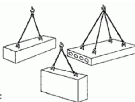
Железобетонные изделия
