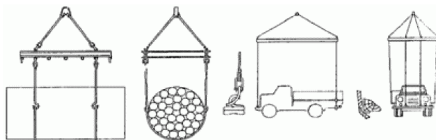
Универсальная траверса для различных грузов
