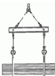
Клещевые захваты для швеллера и рельса
