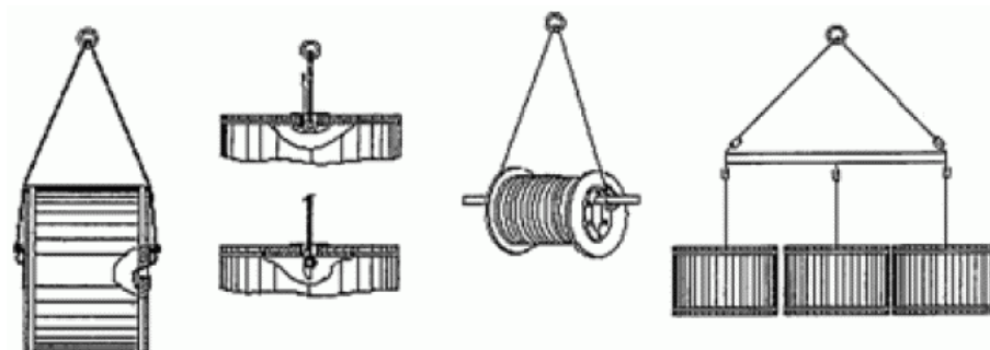
Специальные захваты для барабанов
