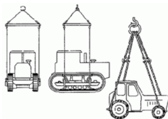
Стропы для тракторов
