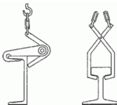
Клещевые захваты для швеллера и рельса
